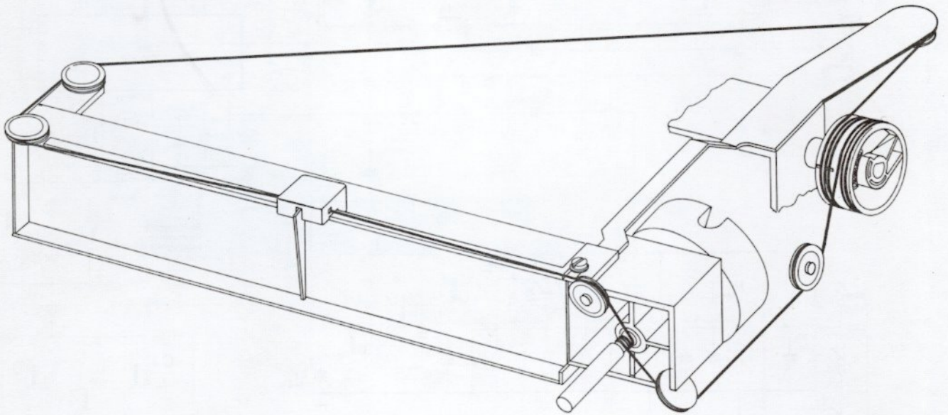
Fig. 5 Seillaufschema
