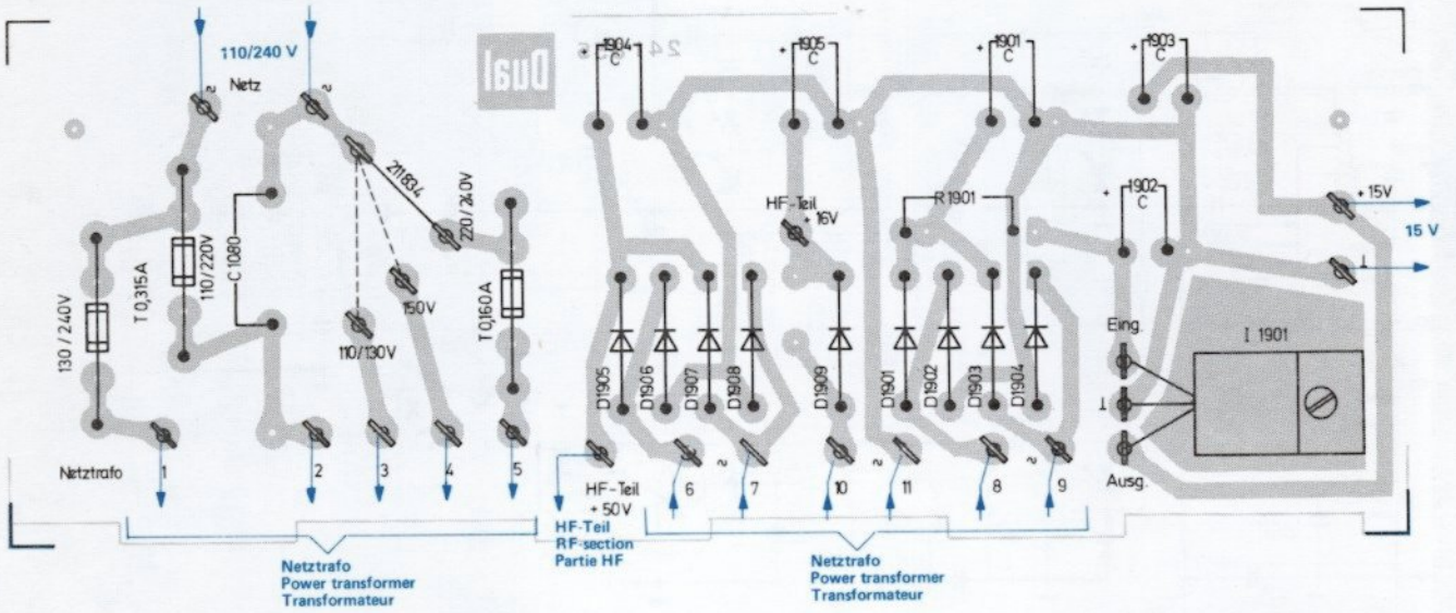
Fig. 4 Stromversorgung Bestückungsseite
