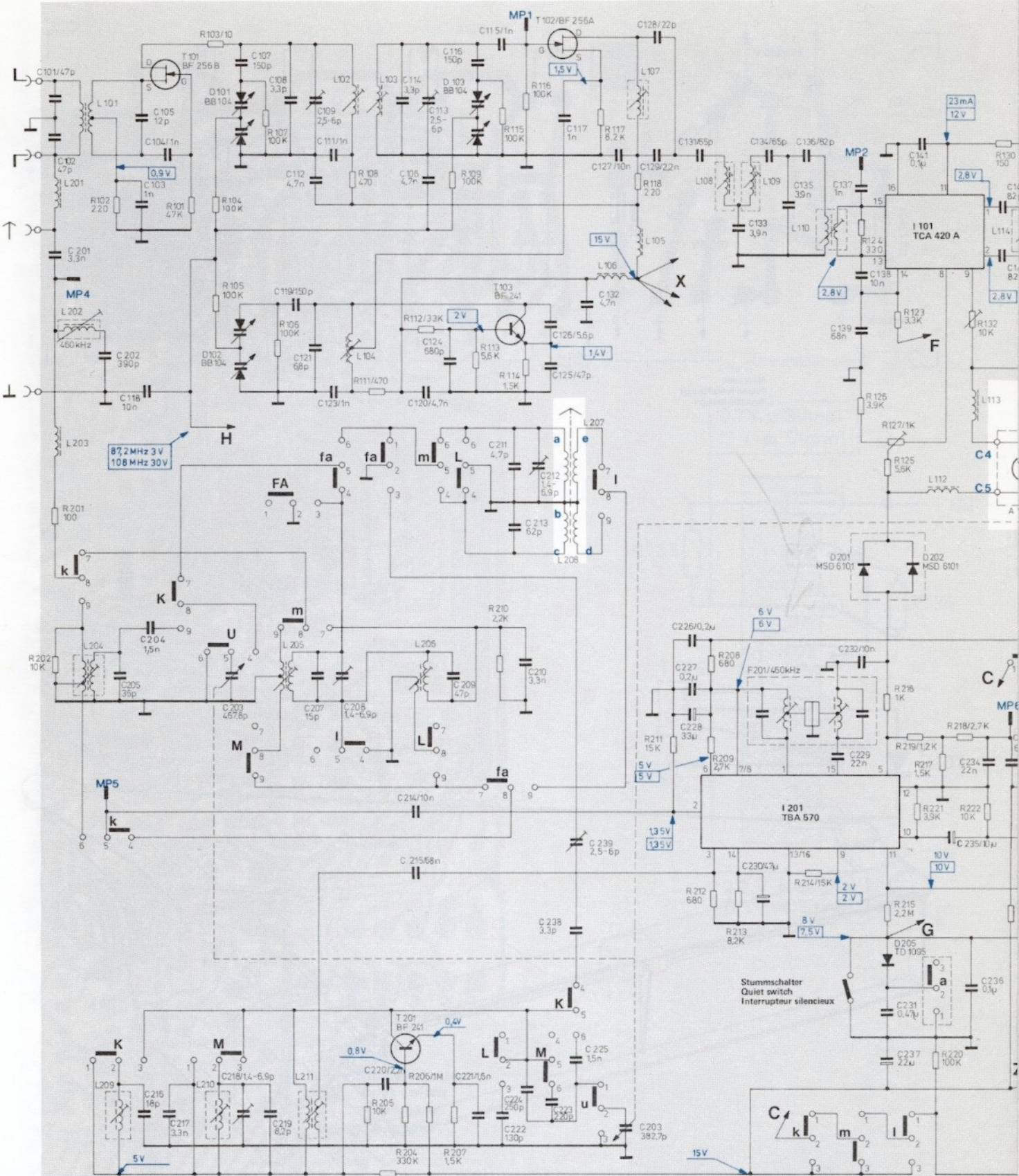
Fig. 2 Schaltbild
