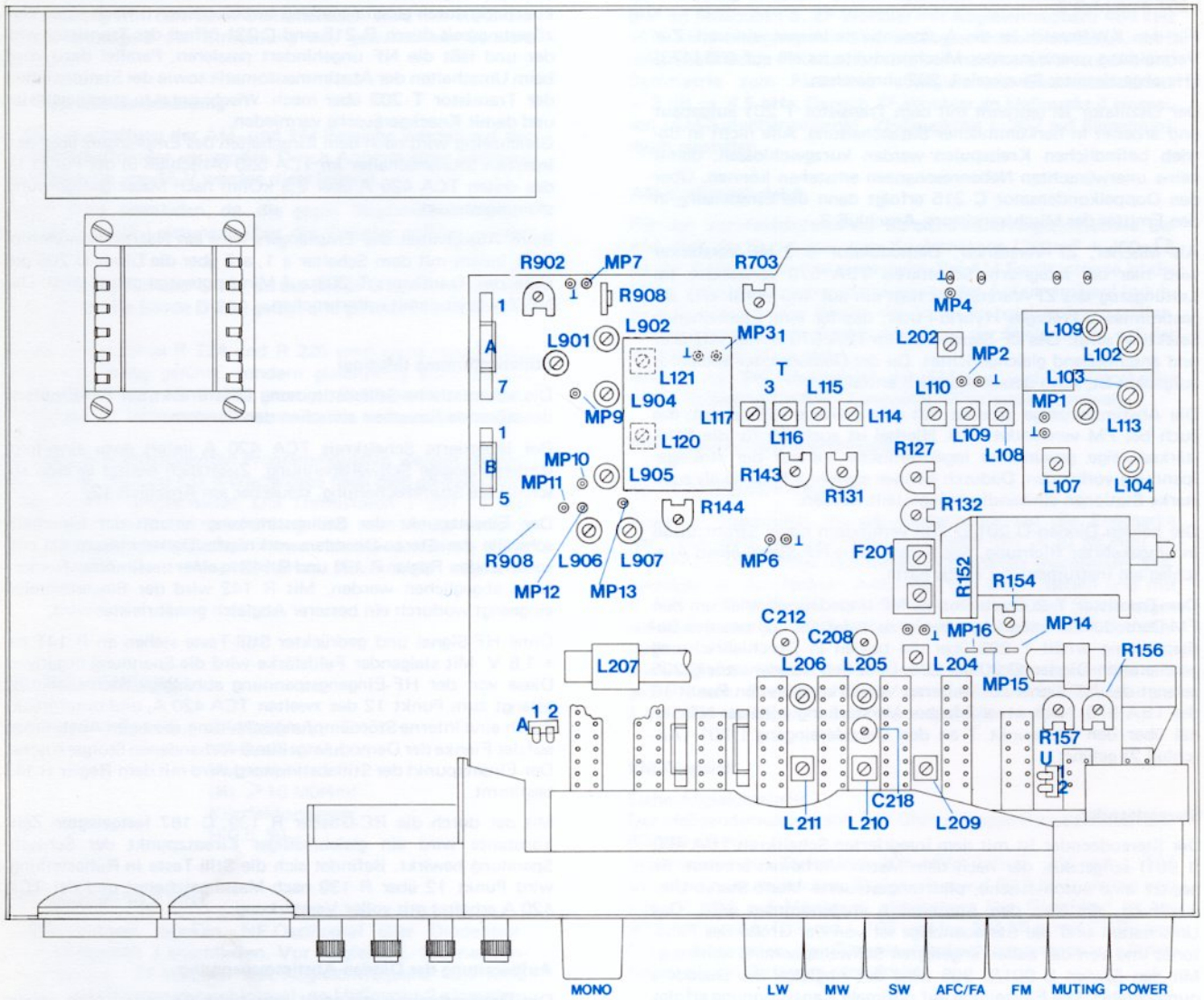
Fig. 1 Abgleichpositionen
